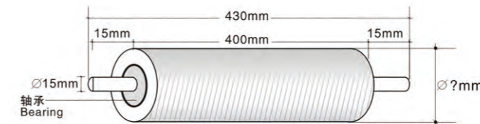
结构示意图 Structure Drawing
